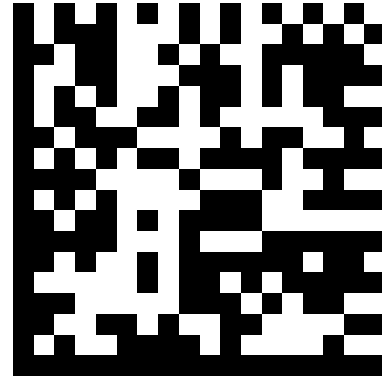
Enable [1]
